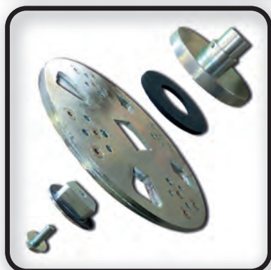
Système de fixation porte-outils avec absorbeur de vibrations
