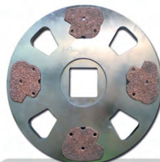
Plateau porte-outils avec segment en carbure
